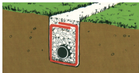
配水管周辺の排水養生
